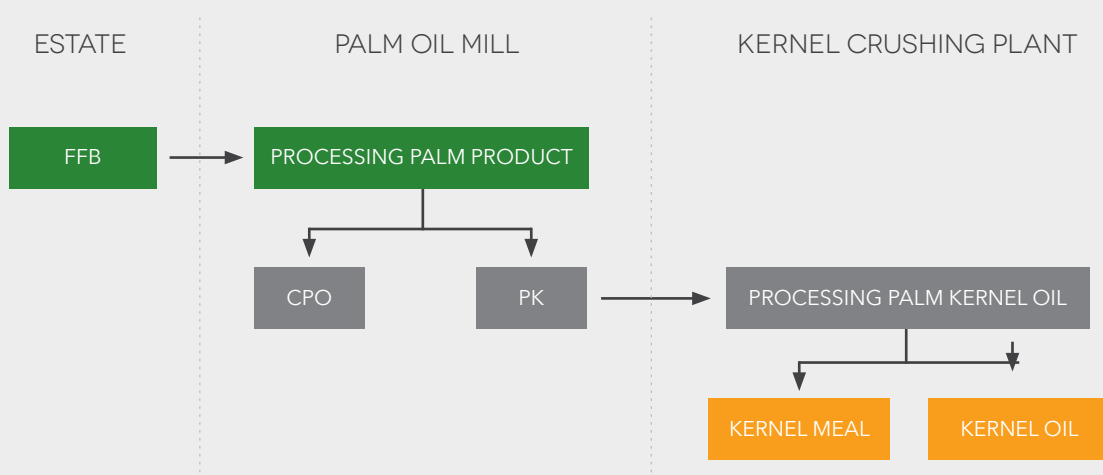
Diagram Proses Produksi Produk-Produk Berbasis Kelapa Sawit
